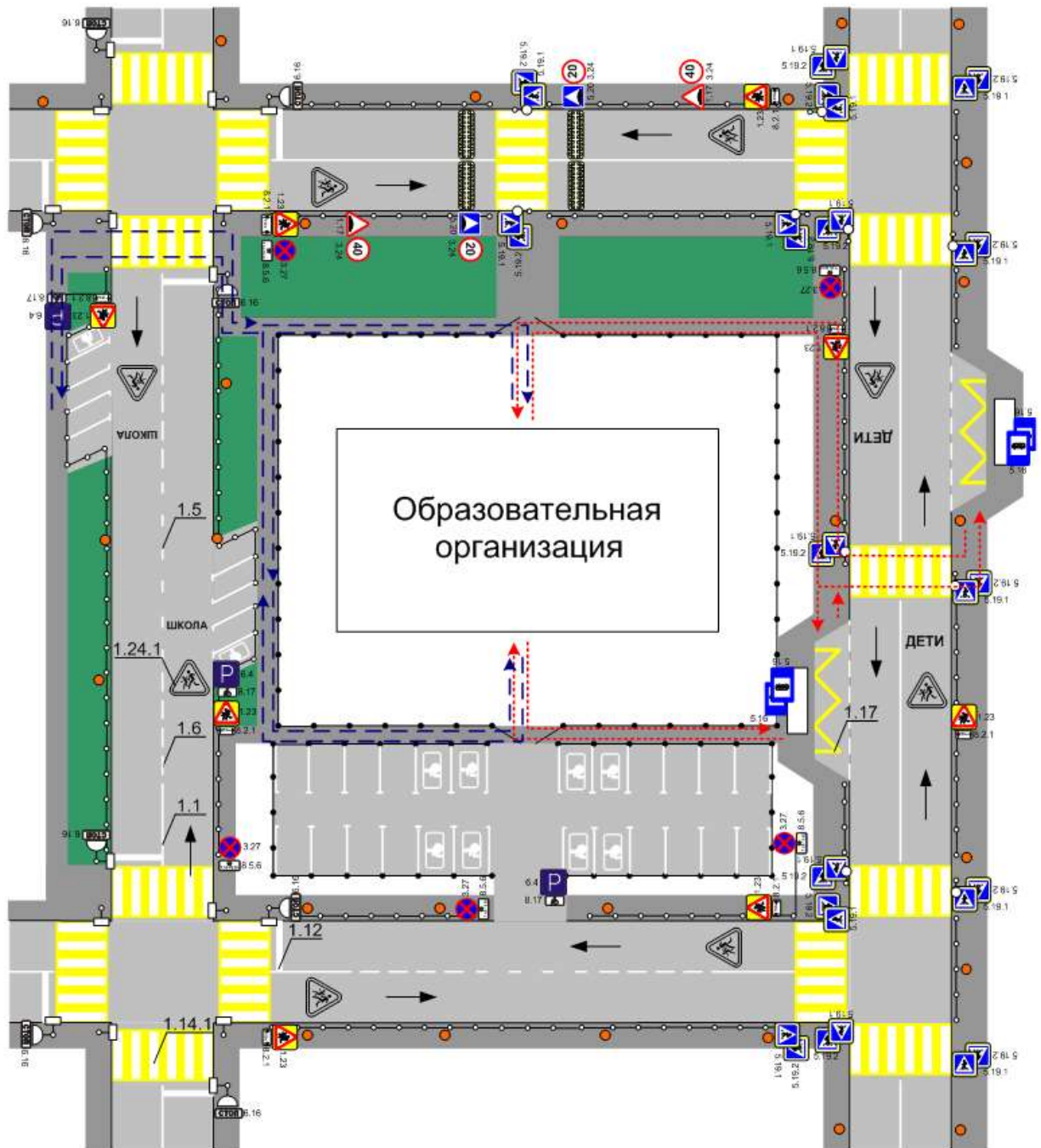
Схема организации дорожного движения около образовательной организации
